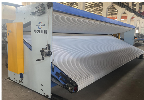
料卷自动喂入系统
